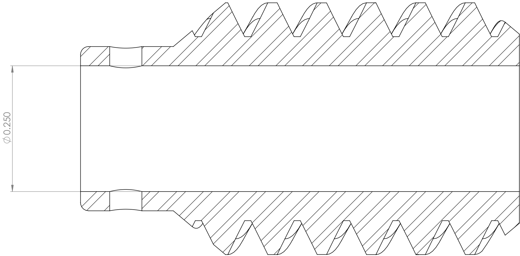
SECTION A-A SCALE 10 : 1
